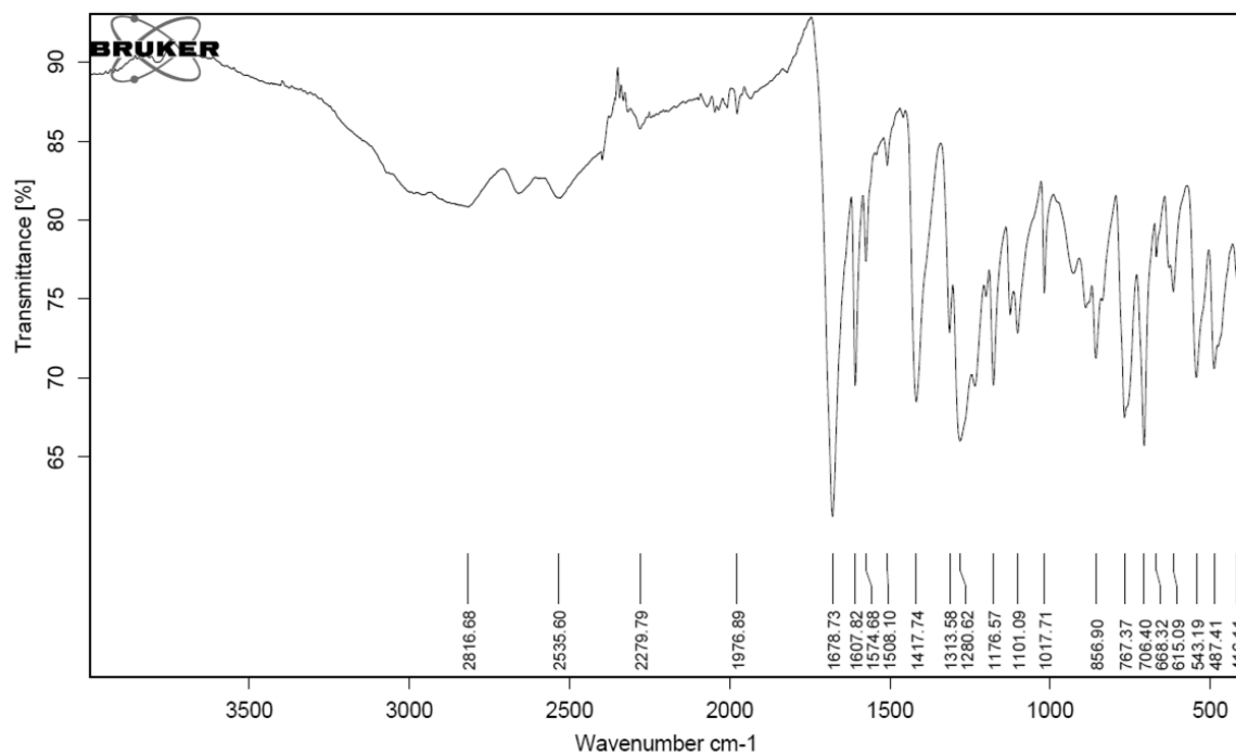
Figure S10. IR spectra of L.
