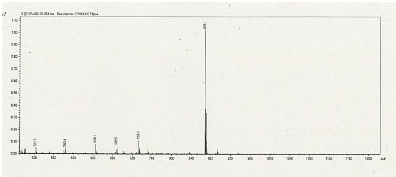
Figure S8. LRMS of L.
