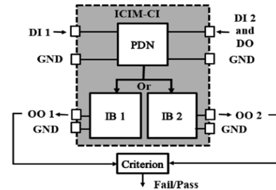
Fig. 1. Dual port ICIM-CI model structure of an IC (Airieau et al., 2016).
