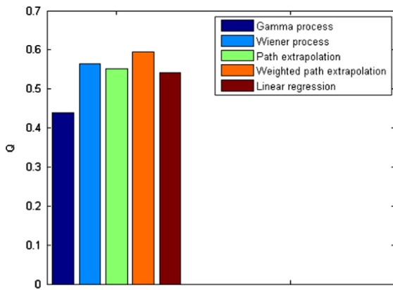
Fig. 5. Mean Q values.
