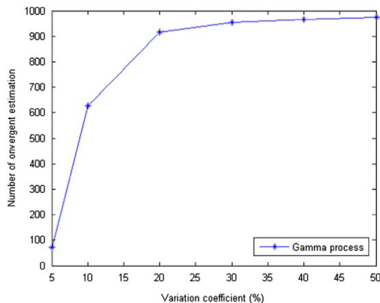
Fig. 12. Number of convergent parameter estimations.
