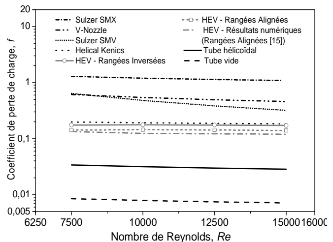
Figure 8 : Coefficients de perte de charge pour des échangeurs de chaleur commerciaux [15]
