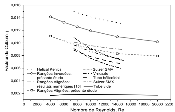
Figure 6 : Facteur de Colburn pour des échangeurs de chaleur commerciaux [15].
