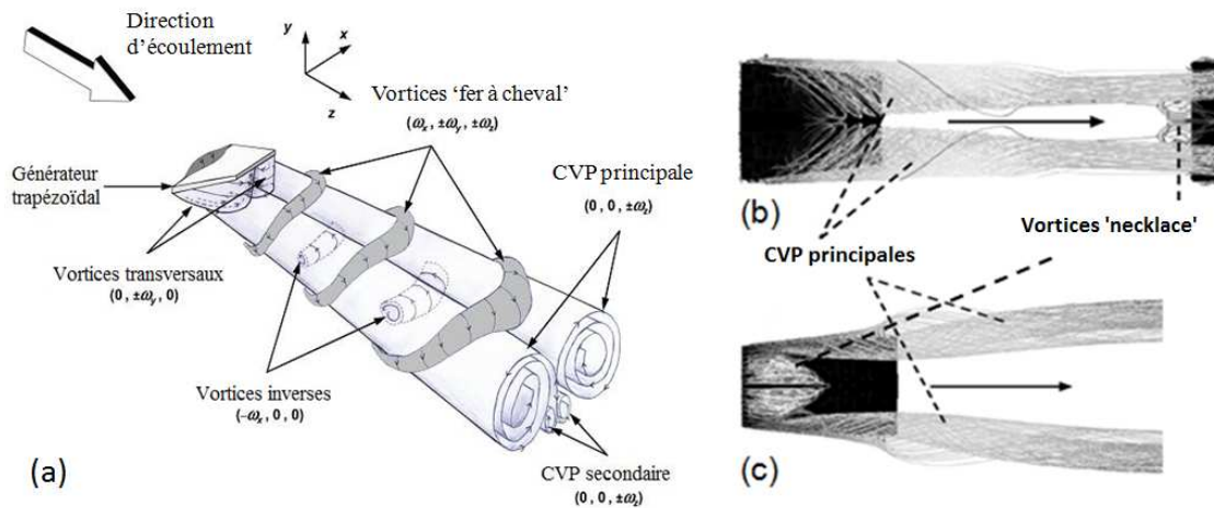
Figure 1 : (a) Structure de l'écoulement produit en aval d'un générateur de vortex trapézoïdal, (b) Lignes de courant – ailettes alignées, (c) Lignes de courant – ailettes inversées.
