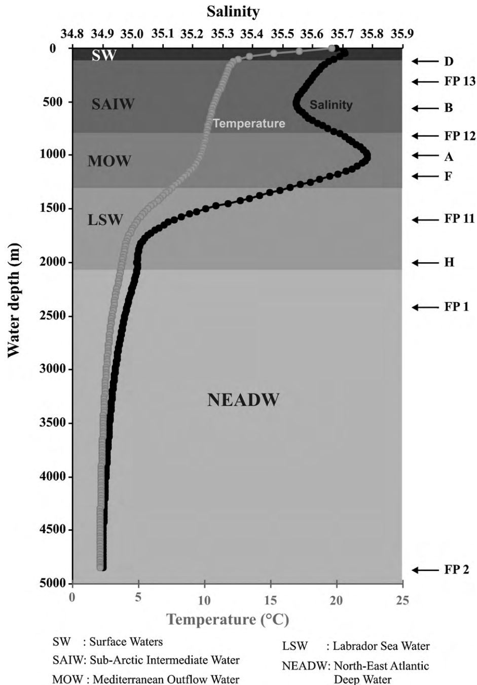
Fig. 2. Salinity and temperature CTD profiles at station FP2 (Van Aken, unpublished data) and the localisation of water masses (After Van Aken, 2000a, 2000b, 2001). Profils CTD de salinité et température à la station FP2 (Van Aken, données non-publiées) et localisation des masses d'eau (d'après Van Aken, 2000a, 2000b, 2001).
