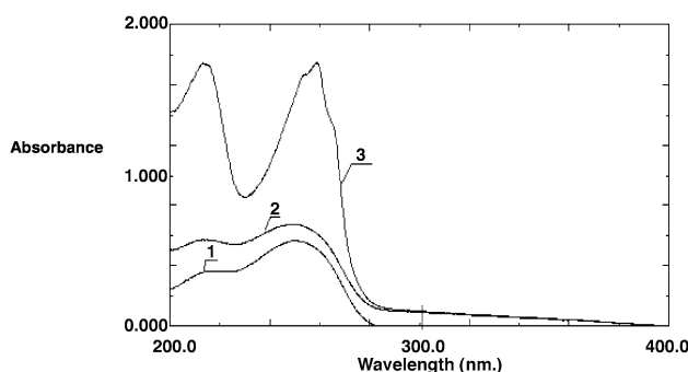
Fig. 3. Absorption spectra of ternary mixtures: 1, KD ( 2 \cdot 10^{-5} \text{ mol l}^{-1} ); 2, KD ( 2 \cdot 10^{-5} \text{ mol l}^{-1} ) + Fe(III) ( 2 \cdot 10^{-6} \text{ mol l}^{-1} ); 3, KD ( 2 \cdot 10^{-5} \text{ mol l}^{-1} ) + Fe(III) ( 2 \cdot 10^{-6} \text{ mol l}^{-1} ) + CPC ( 3.2 \cdot 10^{-3} \text{ mol l}^{-1} ) at pH = 1.6.
